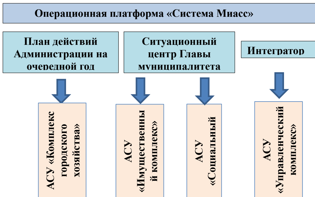
Рис. – Архитектура системы МИАСС
